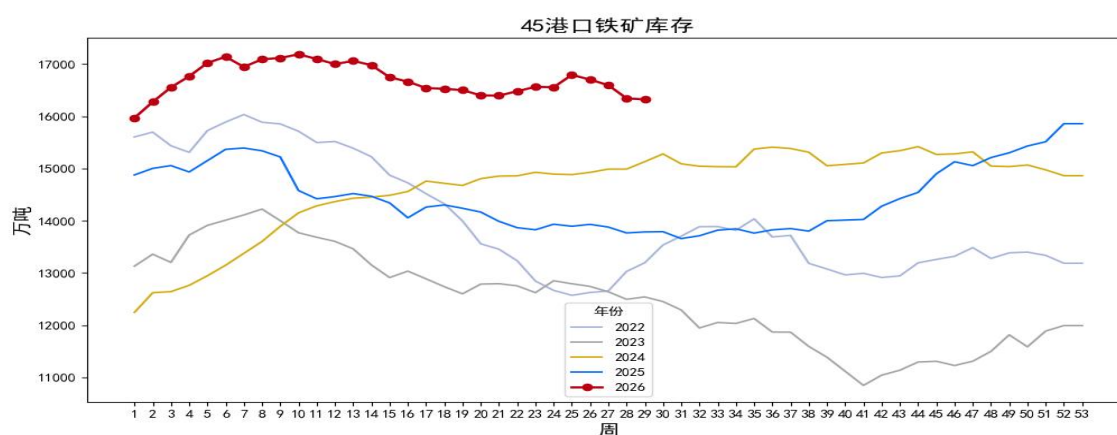
图 10：45 港口铁矿库存
