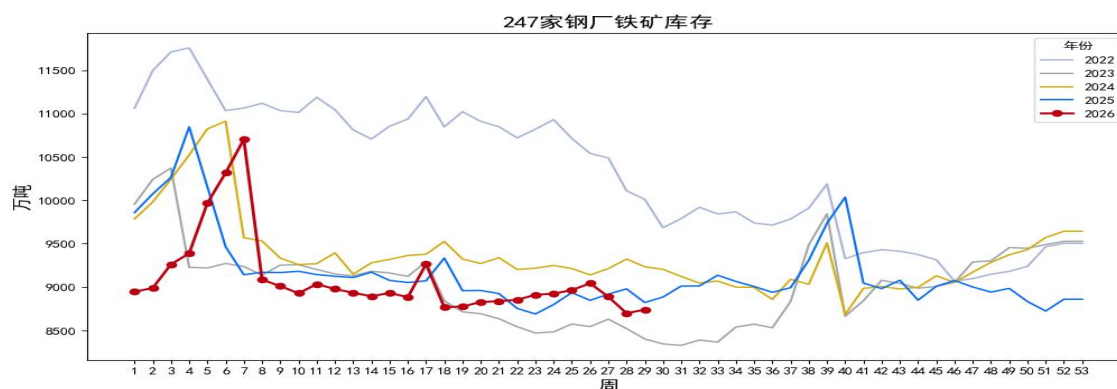
图 9：247 家钢厂铁矿库存
